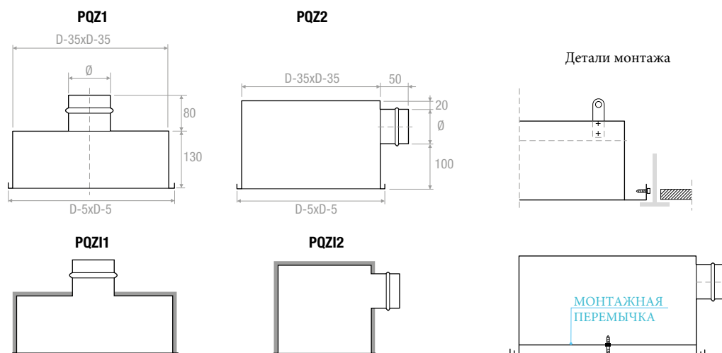
Пленум с наружным утеплением 6 мм
