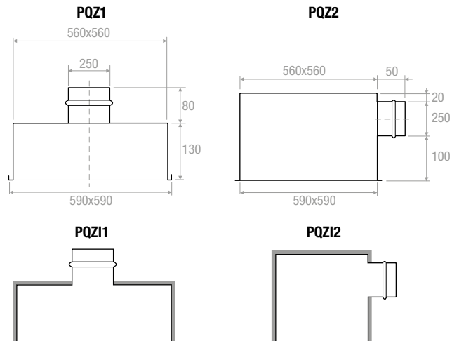
Пленум с наружным утеплением 6 мм
