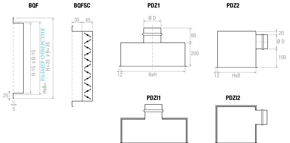
Пленум с наружным утеплением 6 мм
